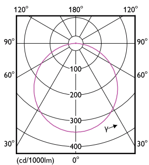
Downlight DN020 G3 NW 14W D150
